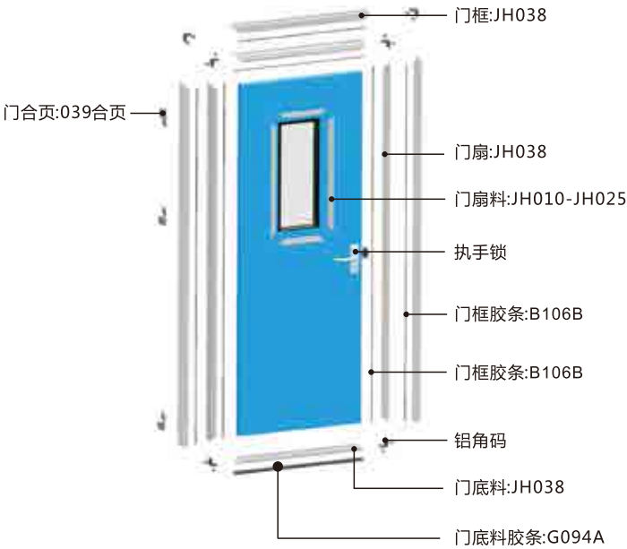
JH038门分解图
