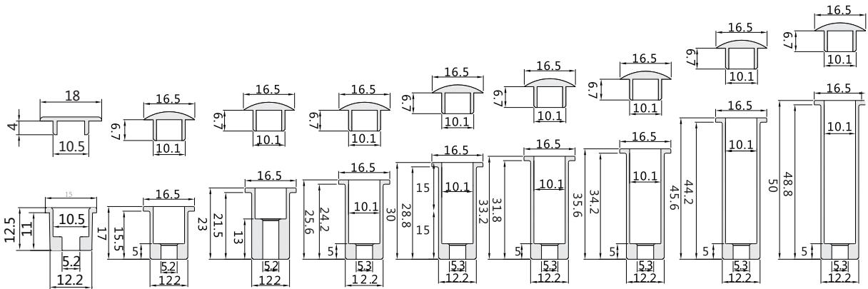
12.5#钉套 17#钉套 23#钉套 25#钉套 30#钉套 32#钉套 35#钉套 45#钉套 50#钉套
